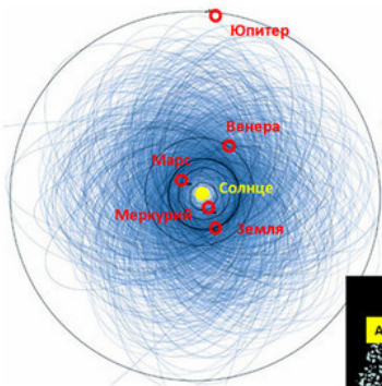
Орбиты потенциально опасных астероидов
