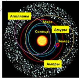
Основные группы околоземных астероидов
