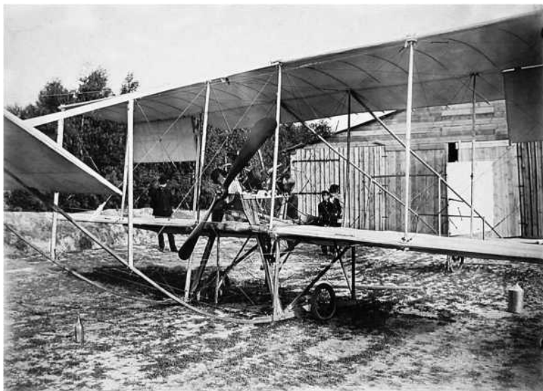
Самолёт «Кудашев-1», 1910 г.
