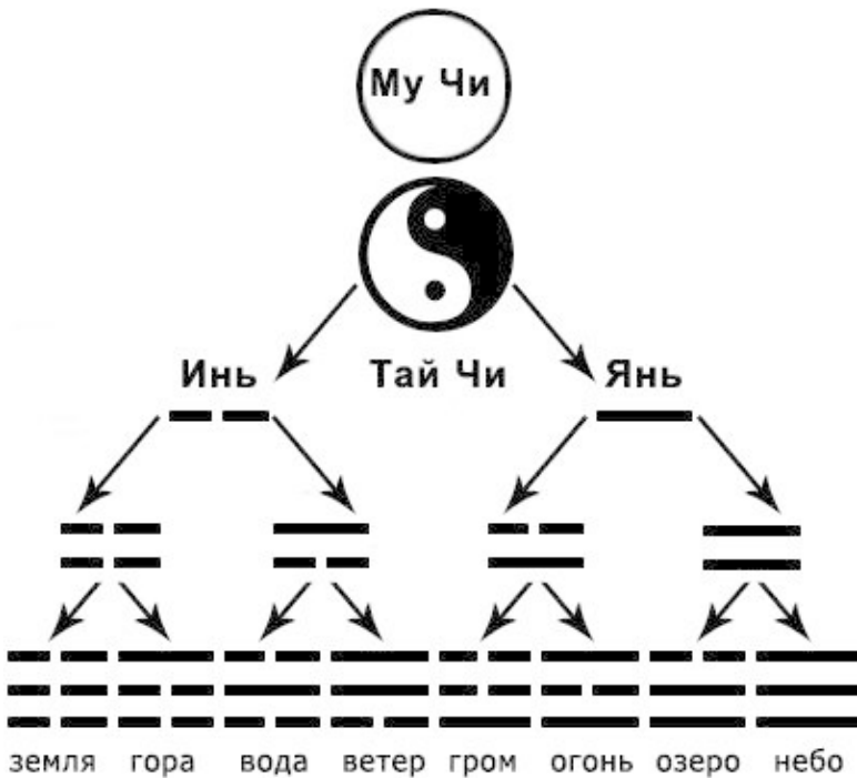
Рис. 4. Формирование триграмм
