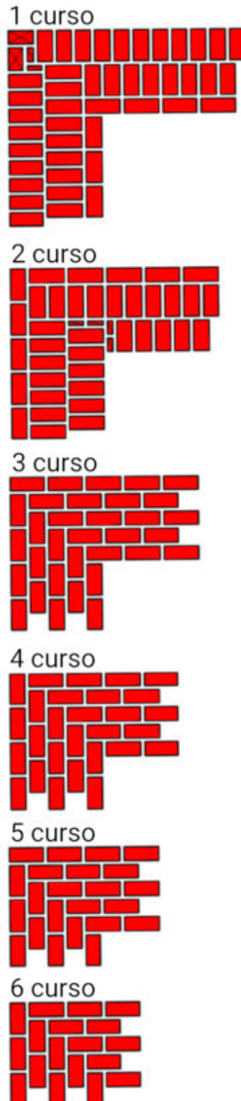
Fig.6. El orden de colocar ladrillos en la esquina de las paredes. Espesor de pared 2.5 ladrillo.
