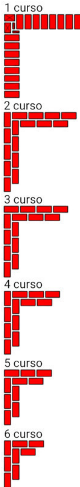
Fig.3. El orden de colocar ladrillos en la esquina de las paredes. Espesor de pared 1 ladrillo.
