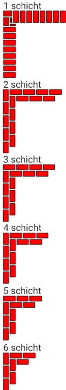
Fig.3. Die Reihenfolge der Ziegel in der Ecke der Wände zu legen. Wandstärke 1 Ziegel.
