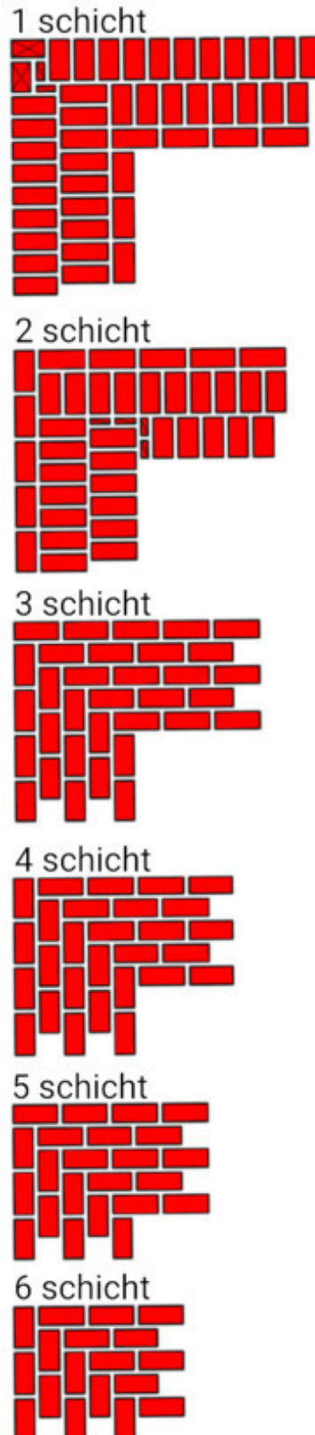
Fig.6. Die Reihenfolge der Ziegel in der Ecke der Wände zu legen. Wandstärke 2,5 Ziegel.
