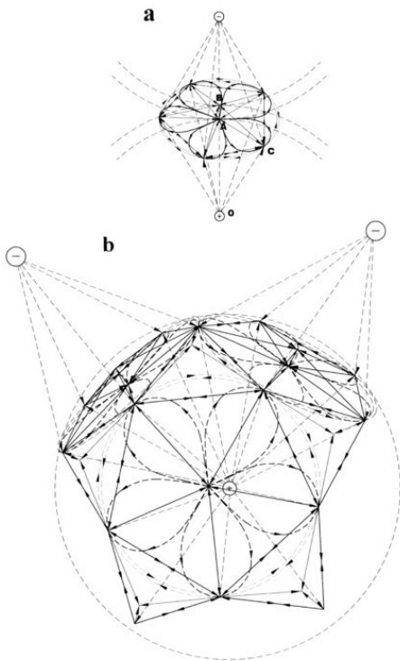
Рис. 22. Динамический (двойные круги встречной циркуляции) и статический (струны) аспекты проявления двой-
