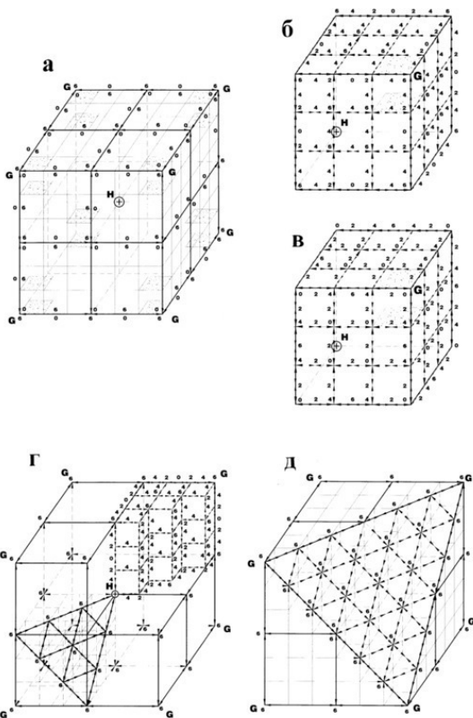
Рис. 11. Распределение единиц потенциалов натяжения и сокращения струн кристаллической решетки гиперкуба Вселенной Света
