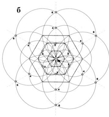
Рис. 32. Сферы истекающего и отраженного Света (а); сферы распространения электромагнитных волн вертикального плана раскрытия луча Света (б)
