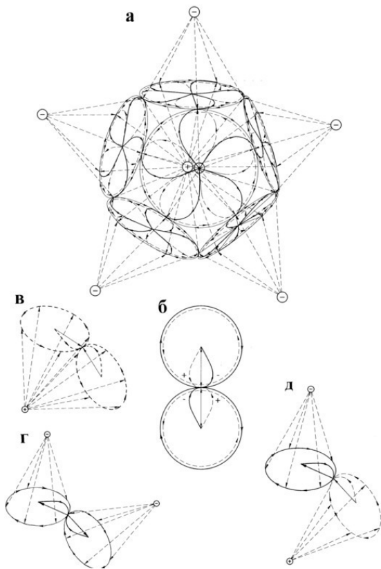
Рис. 27. Циклоническая и антициклоническая циркуляция двойственной силы Света в системе двойных кругов tvoрящих лучей
