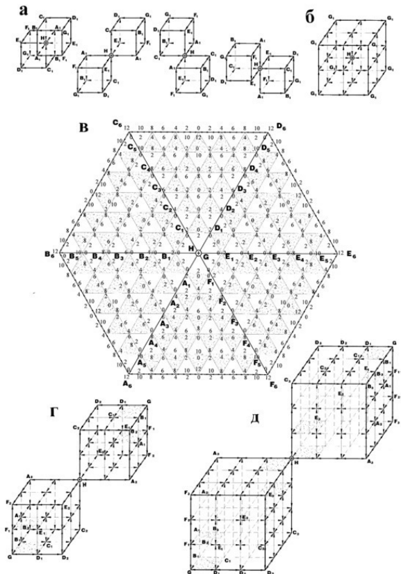
Рис. 10. Моделирование процесса свертки решеток восьми шестиугольников напряжения в кристаллическую структуру гиперкуба Вселенной Света
