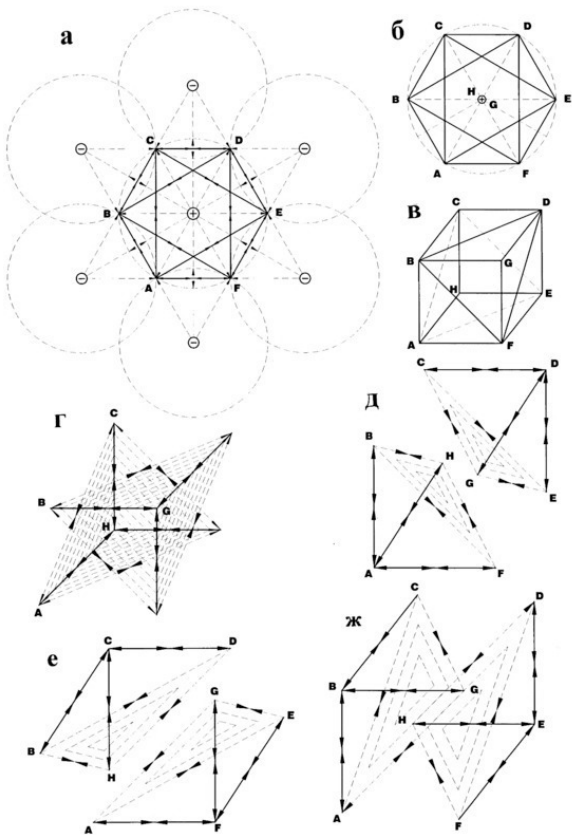
Рис. 8. Моделирование процесса свертки шестиугольника напряжения в один из восьми кубов гиперкуба Вселенной Света
