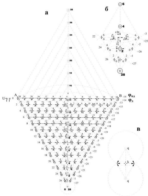
Рис. 4. Распределение единиц потенциала в силовом треугольнике Света
