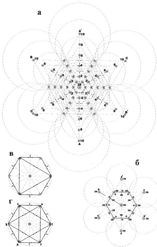
Рис. 6. Фрагмент структуры космической биполярной системы проявления творящей силы Света (двухмерное отображение)
