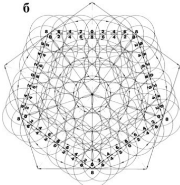
Рис. 33. Резонансная структура распространения электромагнитных волн творящего луча Света с частотой колебания в 1 условную единицу потенциала созидания
