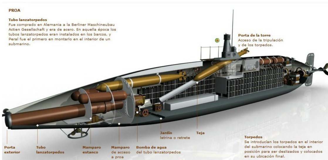
Схема устройства лодки “Peral” (фото El Pais)
