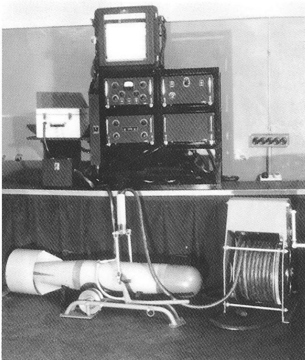
Аэромагнитометр АЭМ-49
