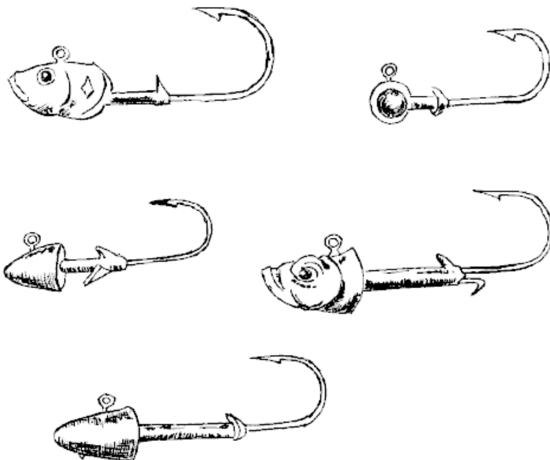
Джиг-головки для силиконовых приманок
