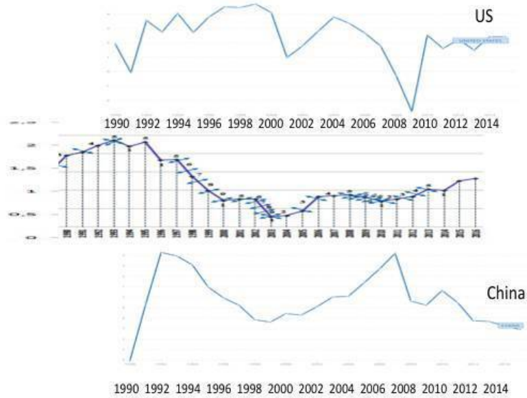
Темпы роста ВВП Китая, США в 1990 – 2015 годах и скорость вращения Земли (LOD) со сдвигом на 4 года
