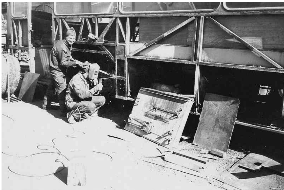
Ремонт Икаруса. 1990
