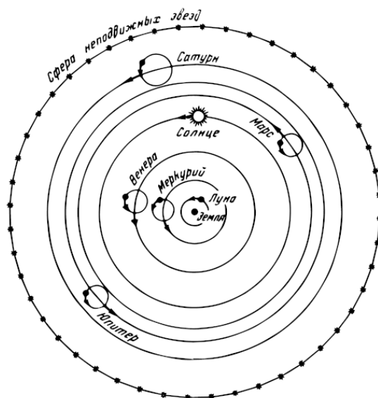
Рис. 4. Система Птолемея. Неподвижная Земля находится в центра мира, планеты движутся по эпициклам, центры эпициклов – по деферентам (орбитам вокруг Земли). У Луны и Солнца эпициклов нет
