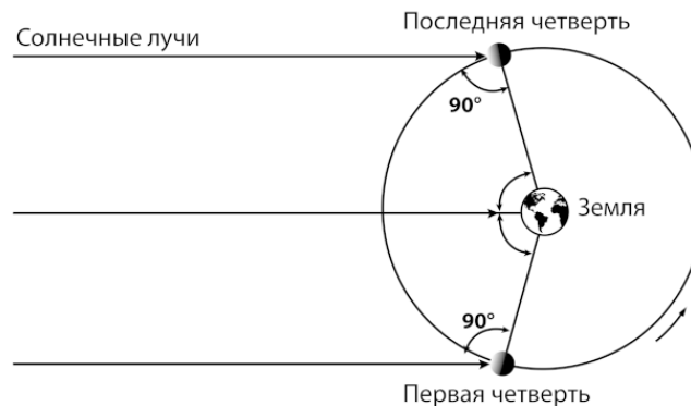
Рис. 3. Определение соотношения между расстояниями до Солнца и до Луны
