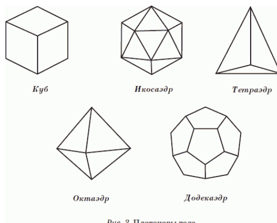
Рис. 3. Платоновы тела
