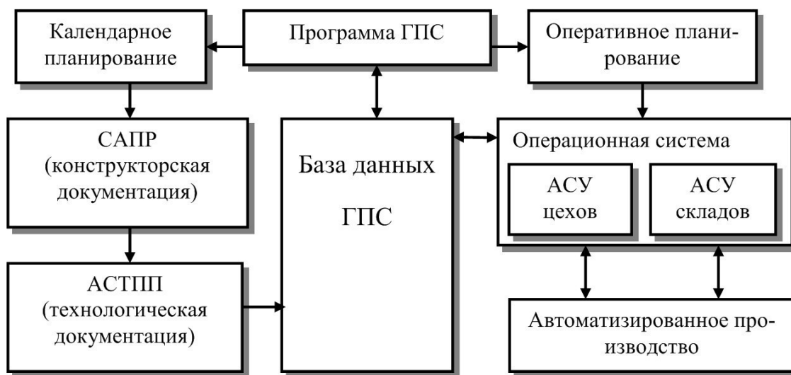
Рис. 1.3. Структура программно-информационного обеспечения ГПС
