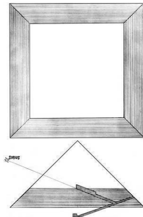
Рис. 9.27. Сечение пирамиды на уровне Камеры Фараона.
