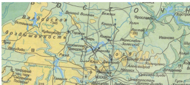
Рис.7. Равносторонний треугольник русских городов: Тверь, Кашин, Дмитров.
