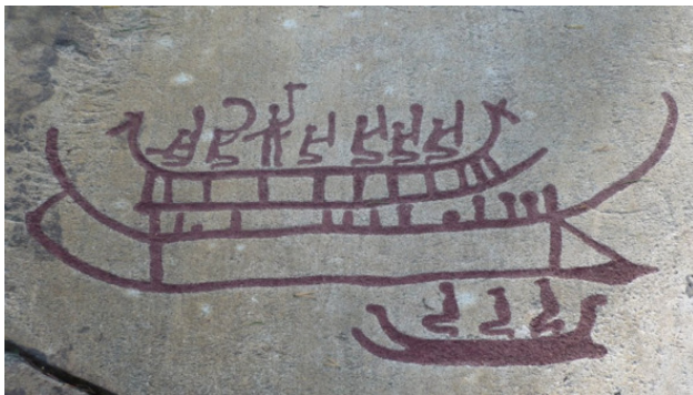
Рис.39. Изображение корабля и его экипажа. Петроглифы. Танума. Швеция.
