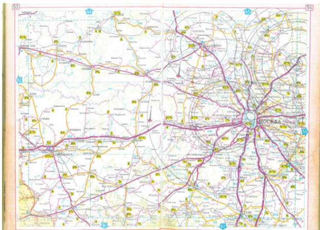
Рис.3. Схема расположения российских городов по кругам-орбитам. Фрагмент карты РСФСР. I регион.// Атлас автомобильных дорог СССР.– М., 1974.
