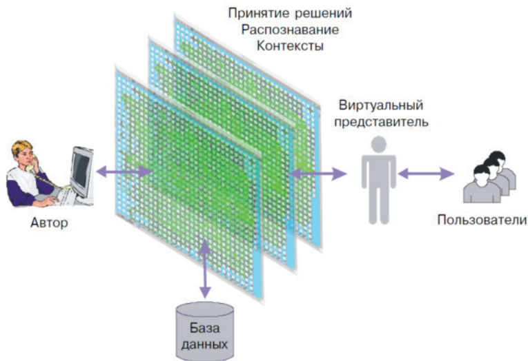
Рис. 2. Виртуальный представитель
