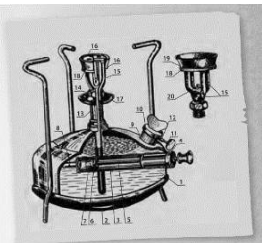
Примус обыкновенный (общий вид) с «шумной» горелкой: 1 – резервуар; 2 – днище; 3 – трубка насоса; 4 – крышка насоса; 5 – шток насоса; 6 – гайка насоса; 7 – кожаный манжет насоса; 8 – клапан насоса; 9 – корпус наливного люка; 10 – крышка наливного люка; 11 – воздушный винт; 12 – трубка воздушного винта; 13 – штуцер; 14 – гайка горелки; 15 – трубчатая часть горелки; 16 – испарительная камера; 17 – чашечка; 18 – упорное кольцо; 19 – отражатель; 20 – форсунка (капсуля, ниппель)
