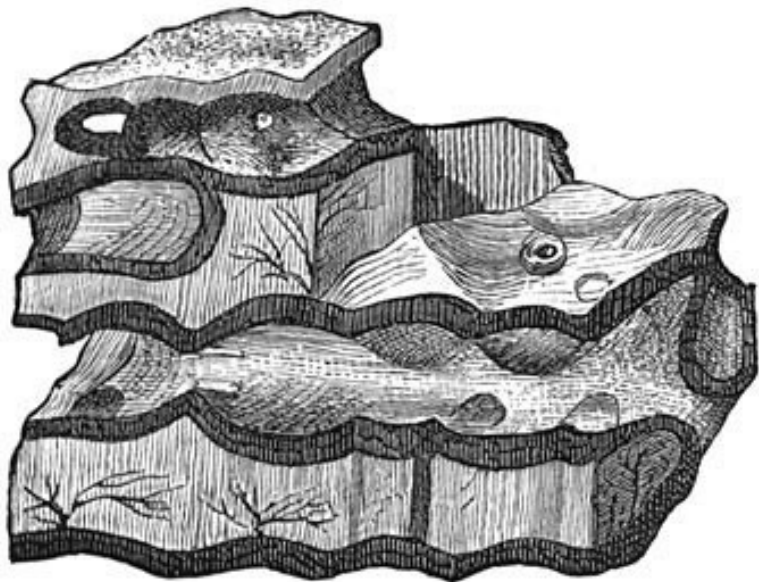
Fig. 65. Oudste bezinkingen. Laurentische formatie. Eozoön canadense .
