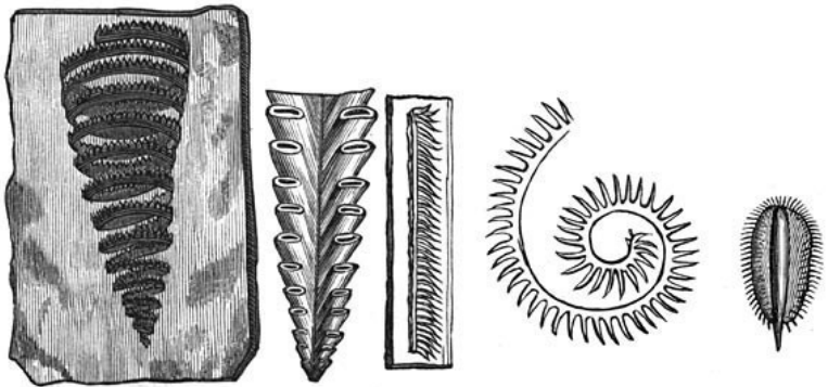
Fig. 73. De oudste dieren. Cambrische periode. Graptolithus turriculatus. Diprion pristis. Monograptus. Bastrites peregrinus. Phyllographtus.
