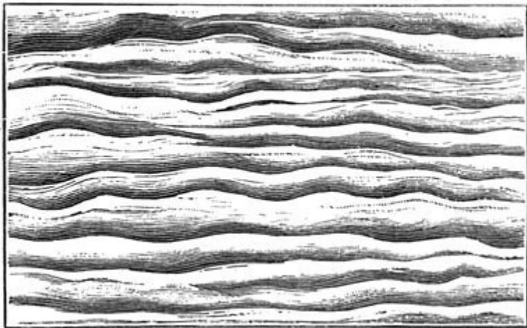
Fig. 15. Versteende golvingen van het water.
