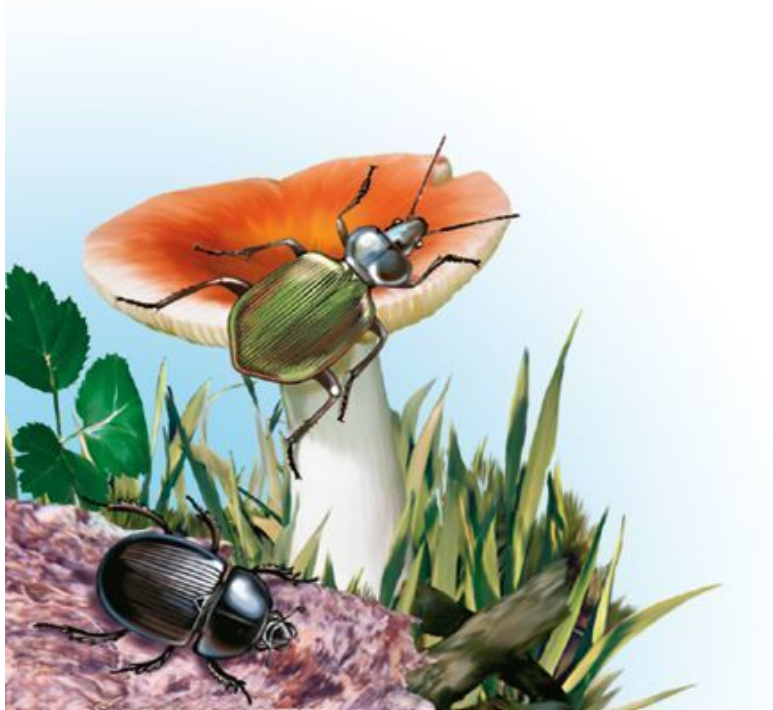
Жужелица (вверху) и навозный жук
