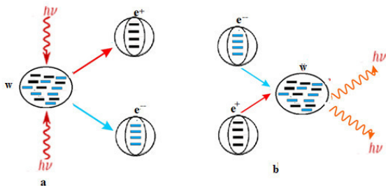
рис. 1. Схема рождения пары частица – античастица
