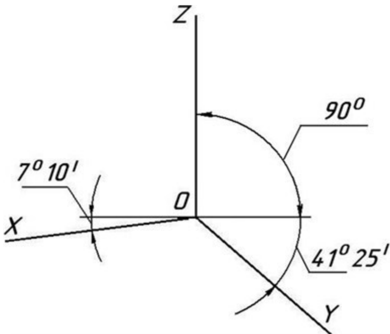
Рис. 12. Расположение осей координат для диметрической проекции
