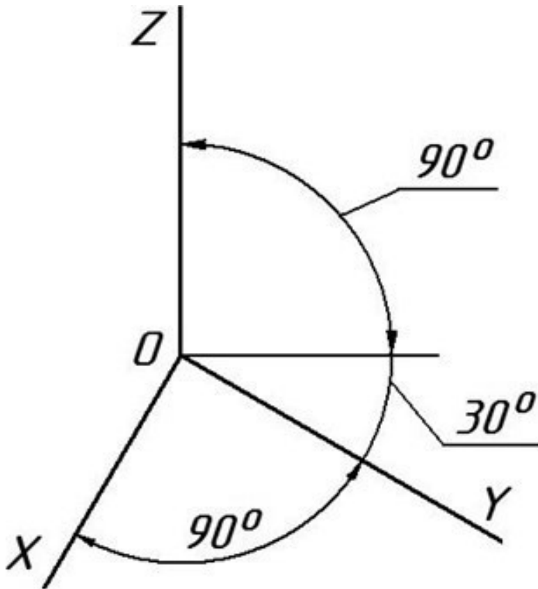
Рис. 14. Оси горизонтальной изометрии
