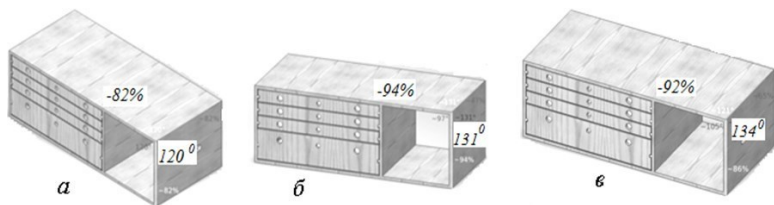
Рис. 10. Виды аксонометрии: а – изометрия; б – диметрия; в – триметрия
