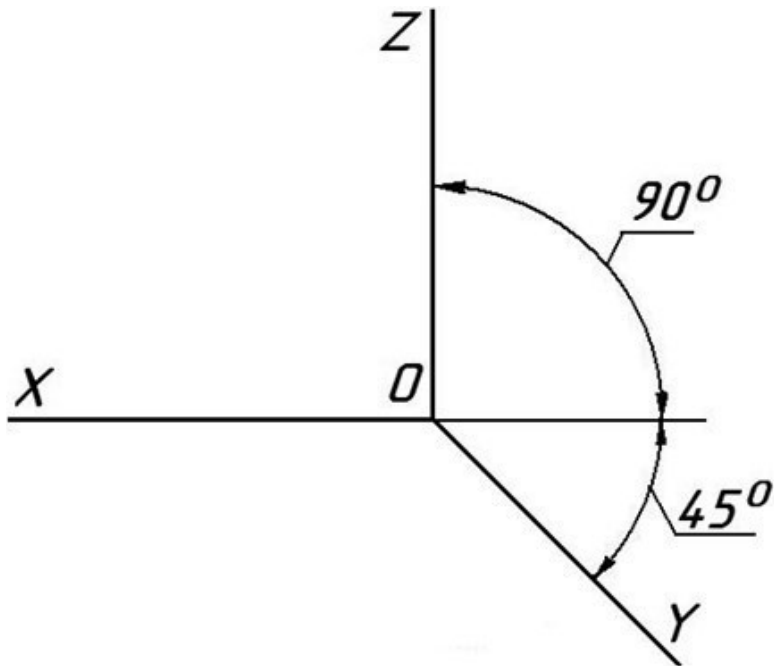
Рис. 13. Расположение осей координат для фронтальной проекции
