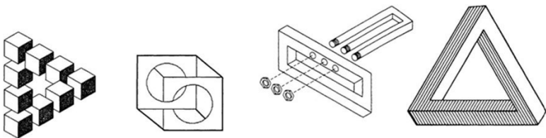
Рис. 7. Невозможные фигуры
