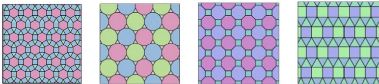
Рис. 6. Полуправильные тесселяции
