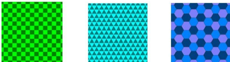
Рис. 5. Правильные тесселяции
