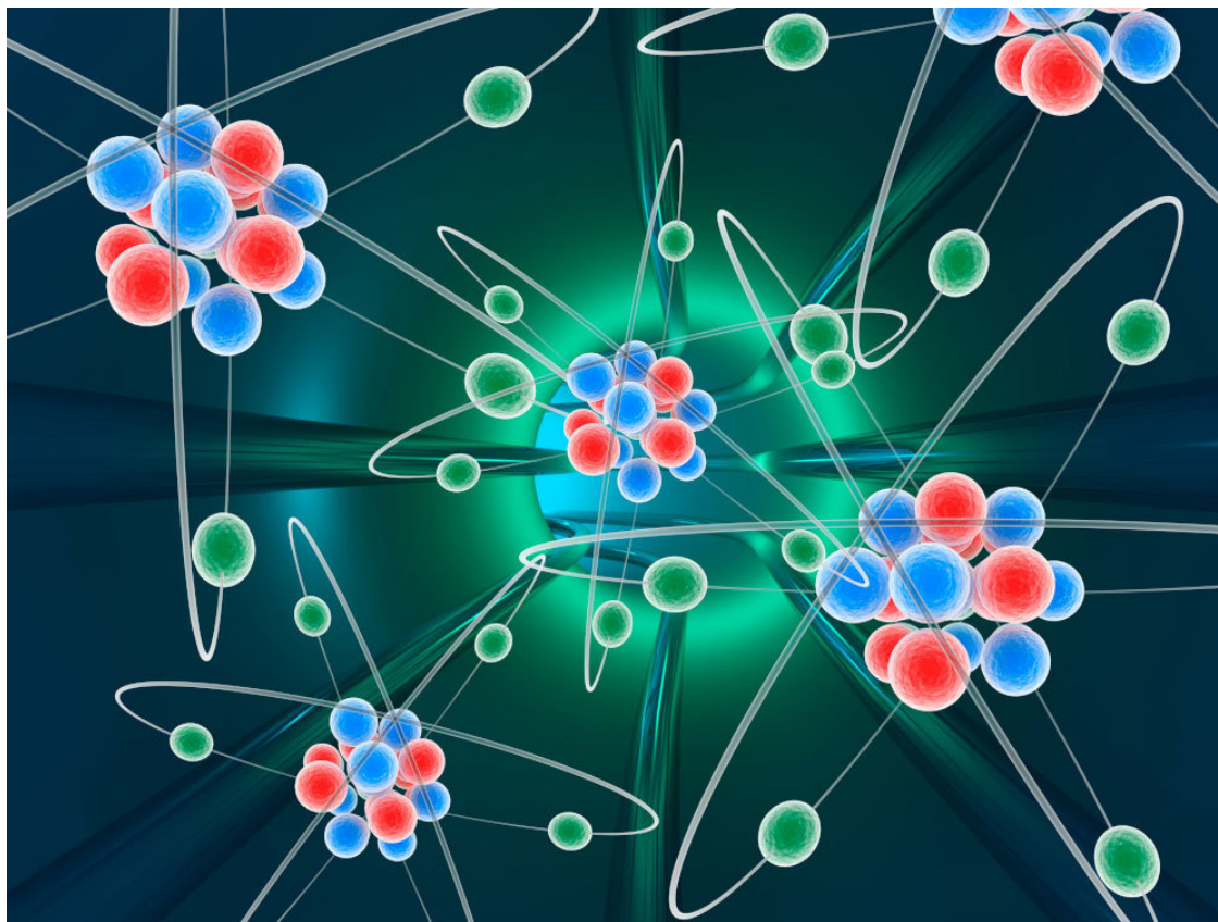
Рис. 9. Структура атома
