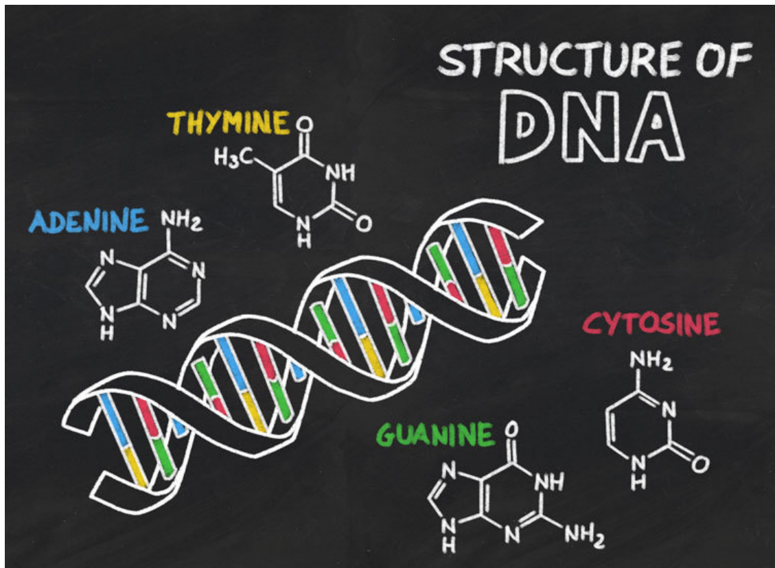
Рис. 6. Структура ДНК
