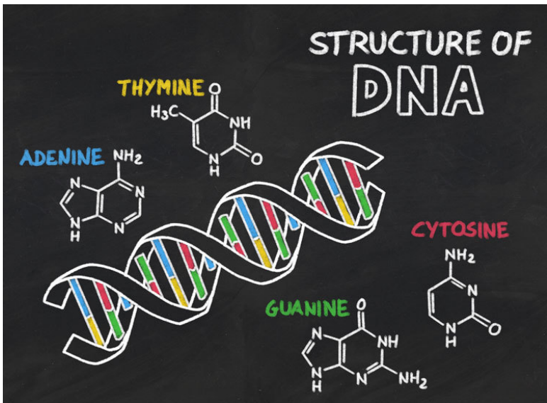
Рис. 6. Структура ДНК
