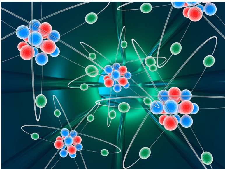
Рис. 9. Структура атома
