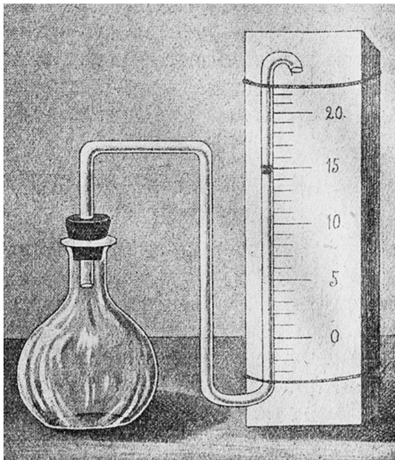
Воздушный термометр
