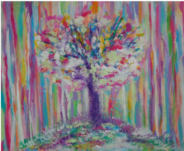
Дерево обновлений (2016)
