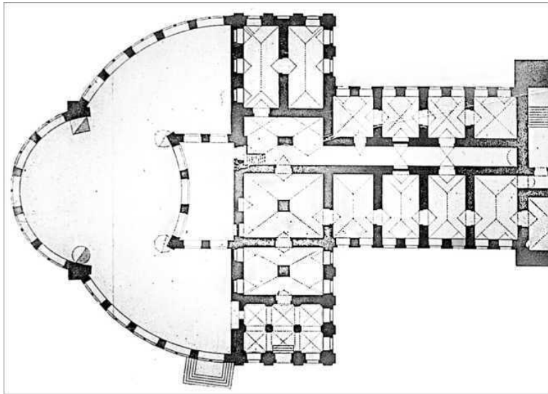
План подвала. Зимний сад с террасой. Фрагмент. Вт. пол. XVIII в.
