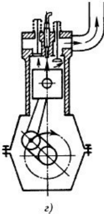
Рис. 3.2.3. Рабочий цикл четырехтактного дизеля: а – впуск, б – сжатие, в – расширение, г – выпуск; 1 — форсунка, 2 — топливный насос высокого давления
