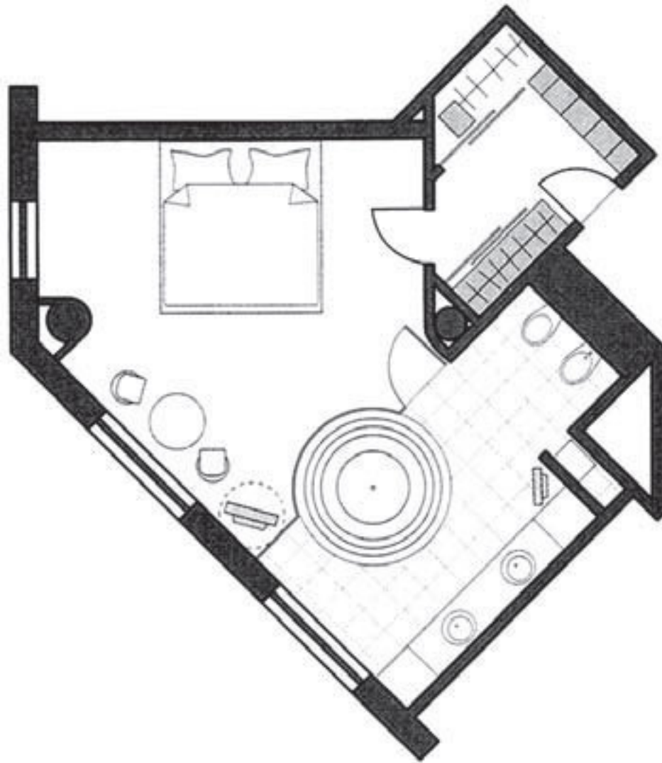
Рис. 2. План зонирования
