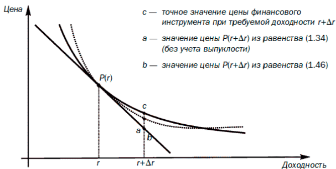
Рис. 1.12. Геометрический смысл основного свойства выпуклости
