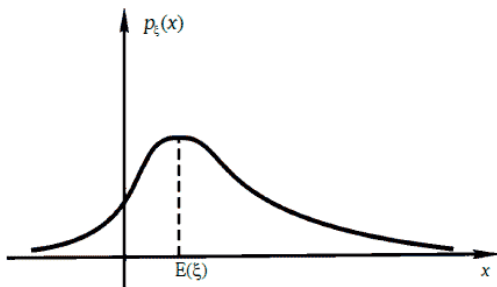
Рис. 1.21. Распределение с правосторонней асимметрией
