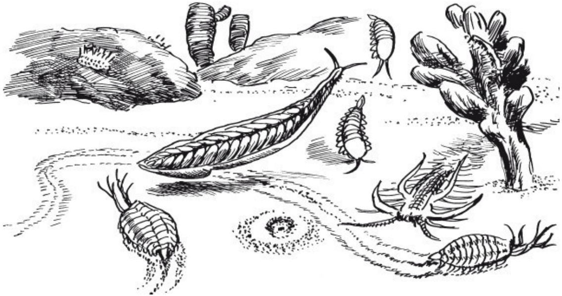
Первое хордовое пикайя
