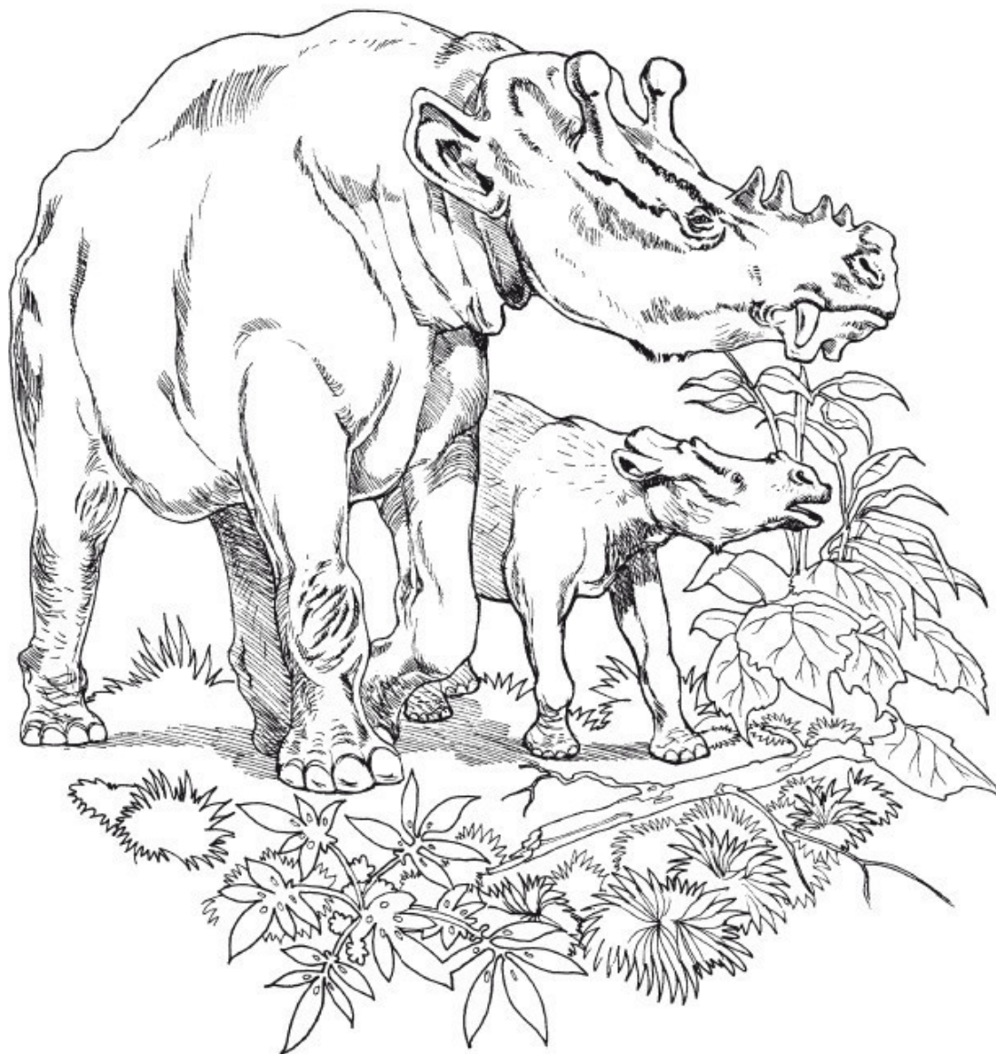
Млекопитающее палеогена – уинтатерий с детенышем
