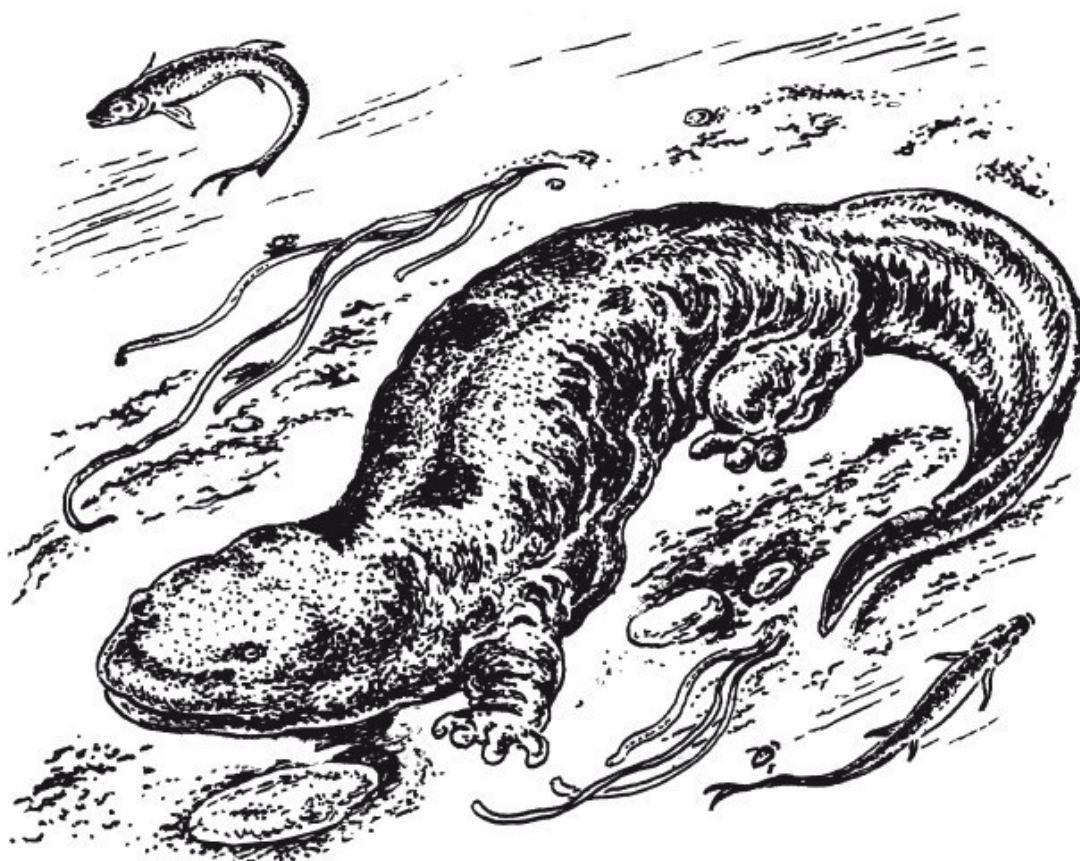
Современная исполинская саламандра
