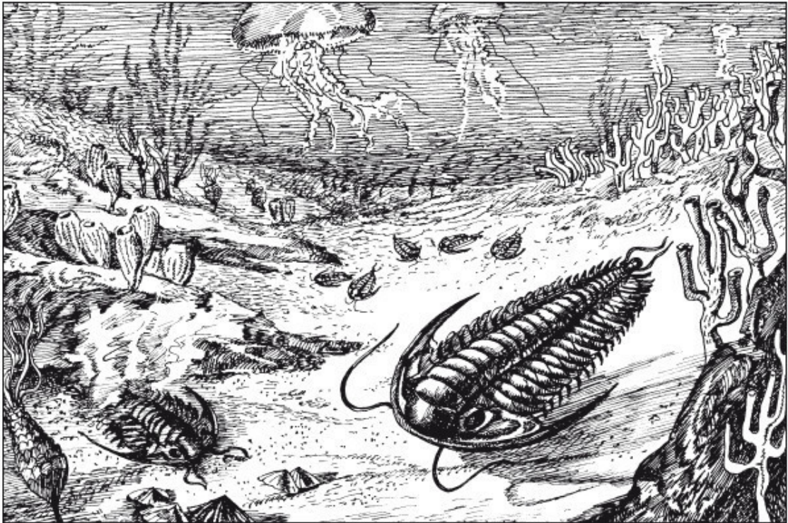
Морское дно кембрия
