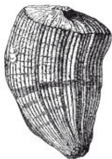
Двустворчатый моллюск Рудист
