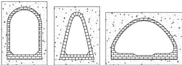
Рисунок 12. Арочные сечения из кирпича и каменных блоков
