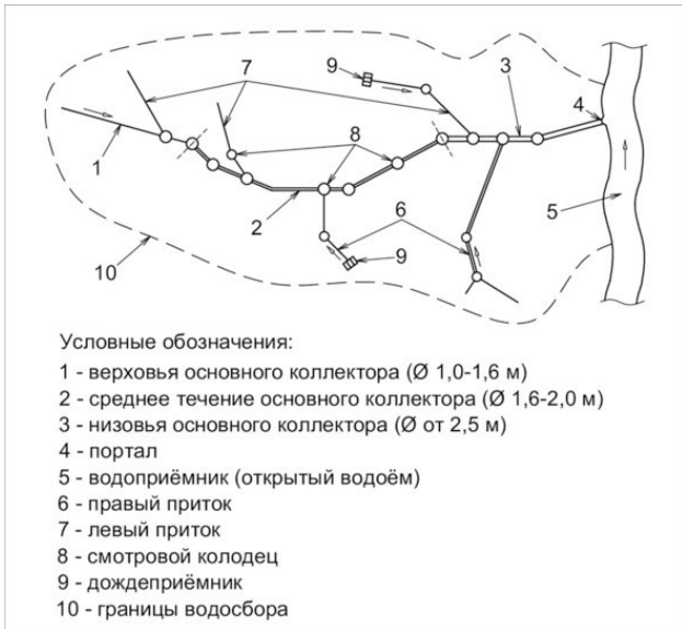
Рисунок 1. Принципиальная схема дренажной сети. Диаметры коллектора указаны для сравнения
