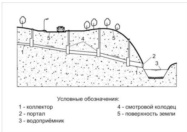
Рисунок 2. Схематичный продольный разрез самотёчного коллектора
