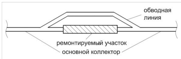
Рисунок 3. Обводной коллектор
