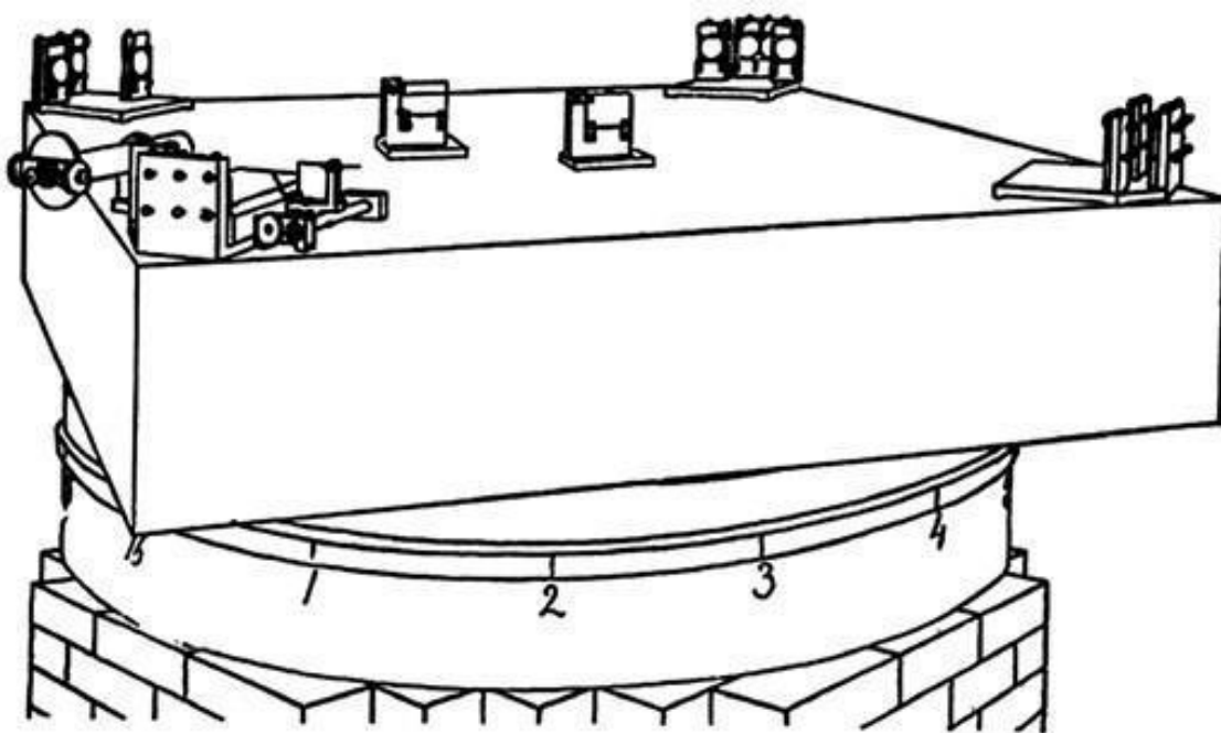
Интерферометр Майкельсона
