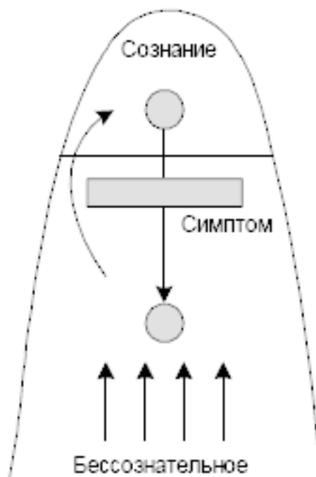
Рис. 3.1. Топическая модель психики. Образование симптома
