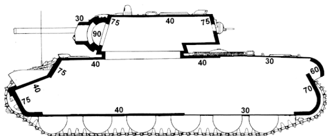
Схема бронирования тяжелого танка КВ-1 выпуска 1940–1941 гг.
