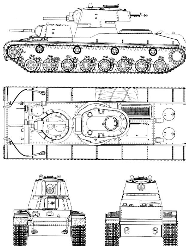
Тяжелый танк СМК. Чертеж В. Мальгинова
