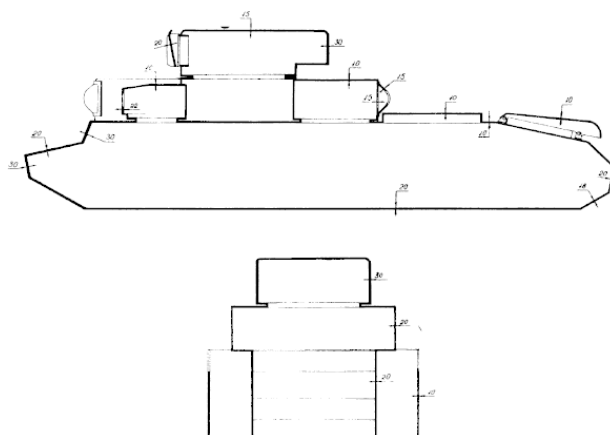
Схема бронирования танка Т-35
