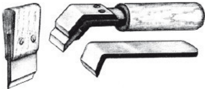
Рис. 1.46. Разновидности циклей
