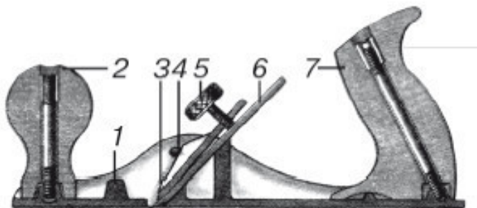
Рис. 1.39. Одинарный металлический рубанок:
