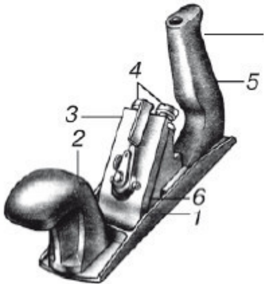
Рис. 1.41. Шерхебель:
