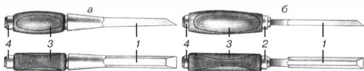
Рис. 1.23. Долото:
