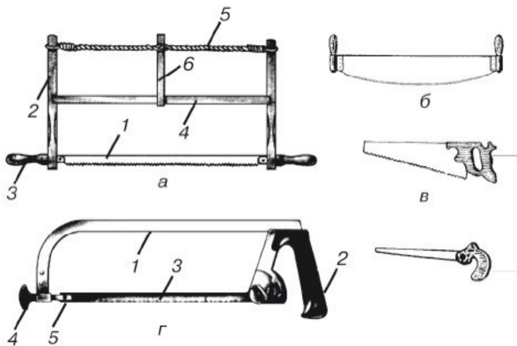
Рис. 1.30. Пилы:
