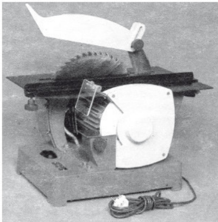
Рис. 1.31. Пила-точило
