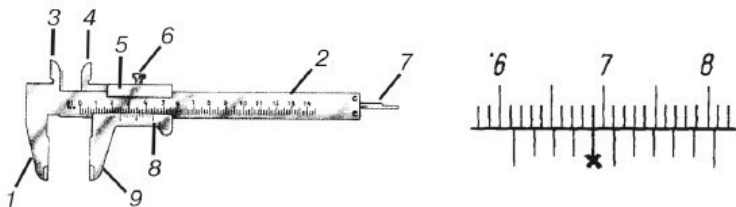
Рис. 1.9. Штангенциркуль:
