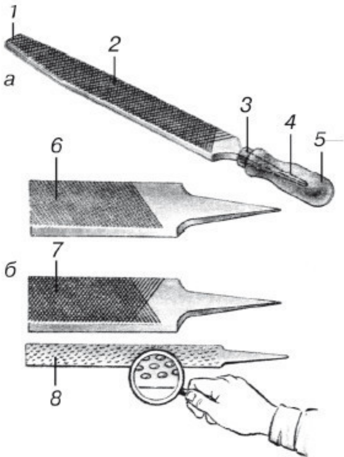
Рис. 1.48. Основные части напильника (а) и виды насе-
