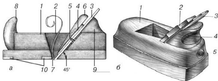
Рис. 1.40. Рубанок с двойным ножом (а) и шлифтик (б): а: 1 – колодка; 2 – ленок; 3 – нож; 4 – стружколом; 5 – винт (крепление стружколома); 6 – клин; 7 – пробка; 8 – рог; 9 – упор; 10 – вставки из твердой древесины; б: 1 – колодка; 2 – клин; 3 – двойной нож; 4 – упор; 5 – пробка
