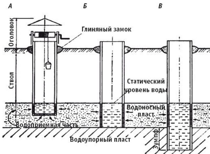
Конструкция шахтного колодца.
