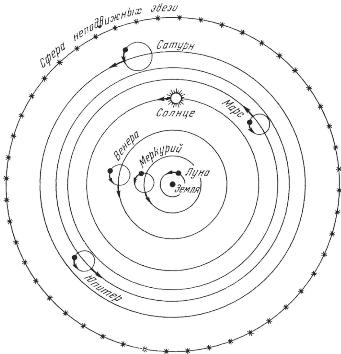
Геоцентрическая система мира
