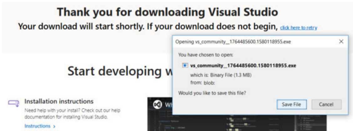
Рис. 2.3. Скачивание веб-установщика
