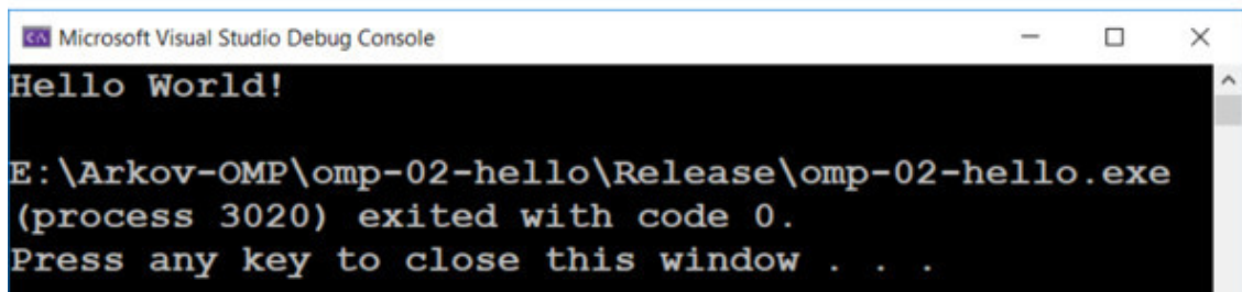
Рис. 3.13. Последовательная программа
