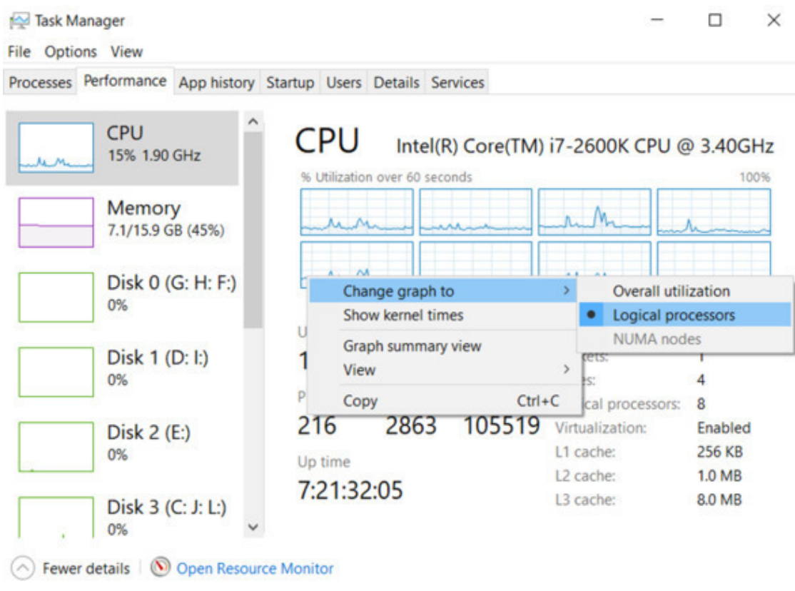
Рис. 3.15. Диспетчер задач
