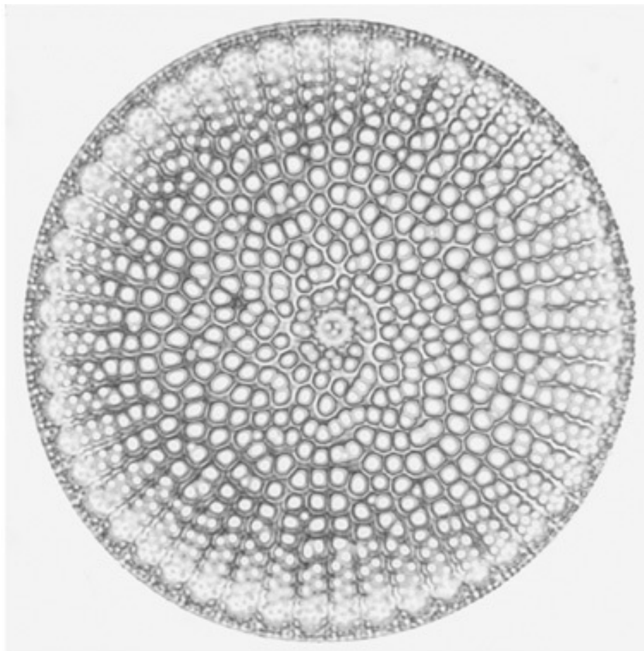
Окаменелые остатки диатомей — одноклеточной водоросли — под микроскопом
