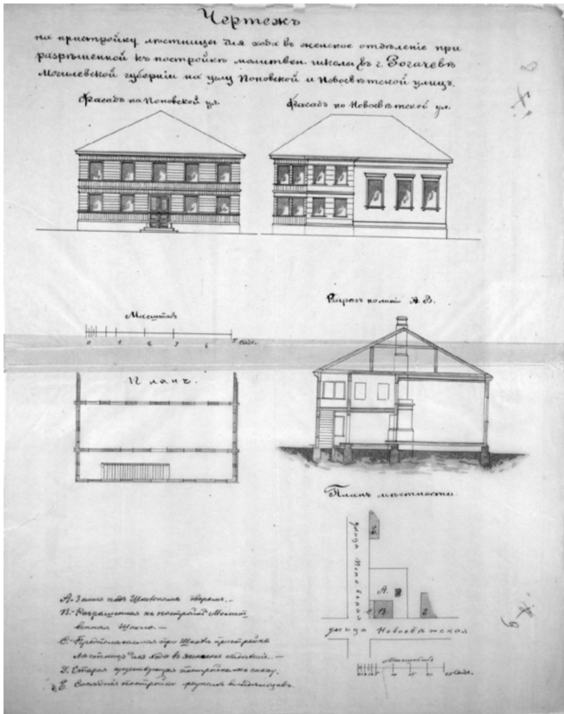
План строительства молитвенного дома на углу Поповской и Новосветской улиц и пристройки к нему лестницы, 1894 г. Источник: http://nashkraj.info/rastsvet-i-upadok-iudejskoj-obshhiny-rogacheva-1850-e-1950-e-gg/
