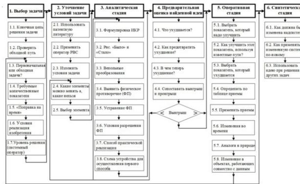
БЛОК-СХЕМА АРИЗ-71В
