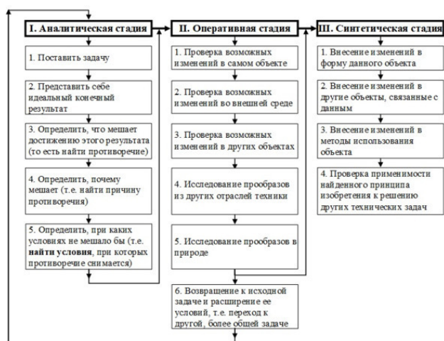
БЛОК-СХЕМА АРИЗ-59
