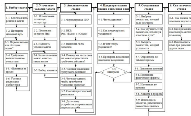
БЛОК-СХЕМА АРИЗ-71
