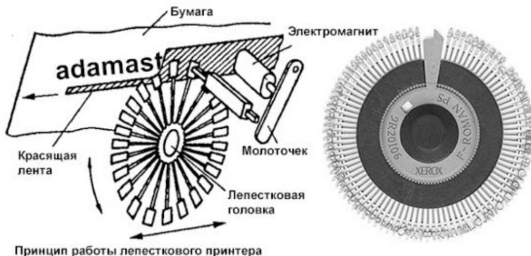
Рис. 3.9. Лепестковый принтер 24
