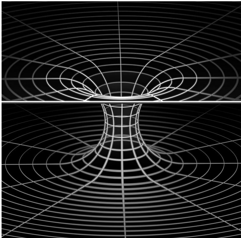
Схема гравитационного коллапса
