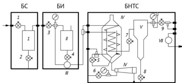
Рис. 8б. Структура блока сепарации (рис. 8а)
