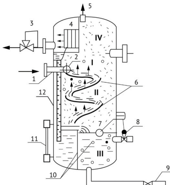
Рис. 8в. Устройство вертикального сепаратора
