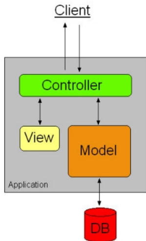
Рисунок 20. Концепция Model-View-Controller
