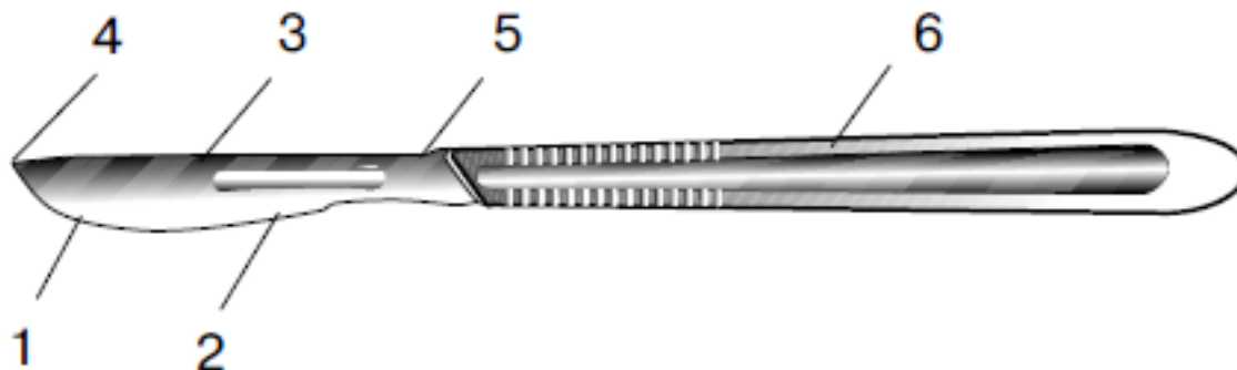
Рис. 23. Части конструкции хирургического ножа (скальпеля): 1 – лезвие; 2 – режущая кромка; 3 – обухок; 4 – кончик лезвия; 5 – шейка; 6 – ручка (по: Medicon instruments, 1986).
