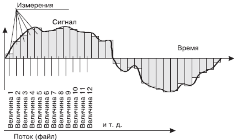
Рис. 1.5. Принцип оцифровки аналогового сигнала
