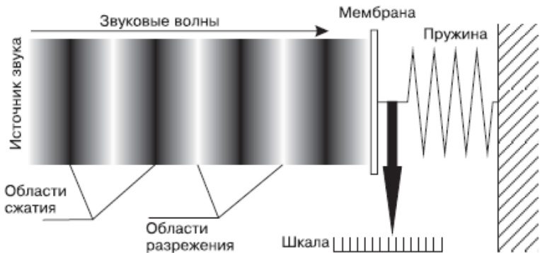
Рис. 1.1. Звуковые волны и звуковое давление
