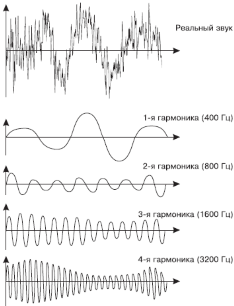
Рис. 1.4. Разложение колебания на гармонические состав-
