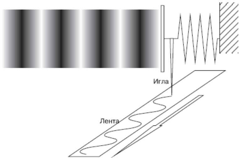
Рис. 1.2. Запись звуковых волн
