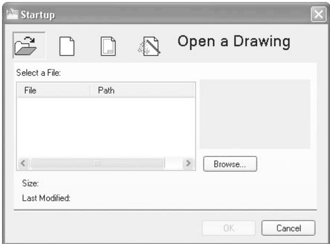
Рис. 1.32. Открытие чертежа
