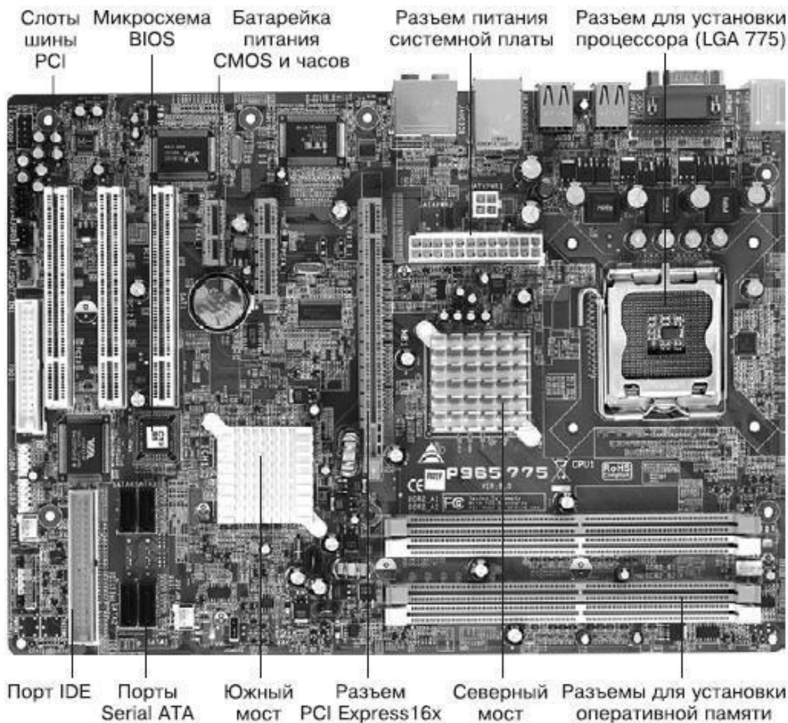
Рис. 1.2. Системная плата
